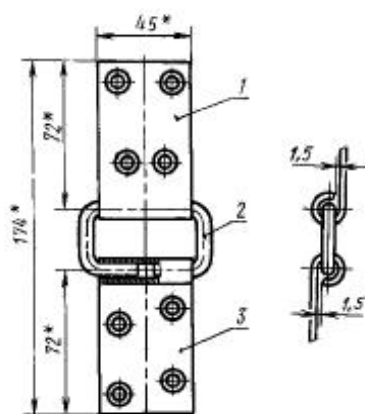
Шарнирная петля 3 ОКП 72898 83401
