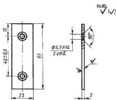
Черт. 27
