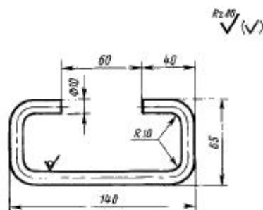
Скоба (для ручки 3)
