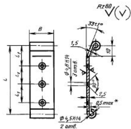
Исполнение 1
