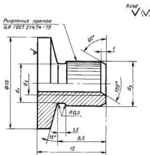
Черт.35
